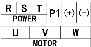
主回路接线端子图(185 ~ 350kW)
