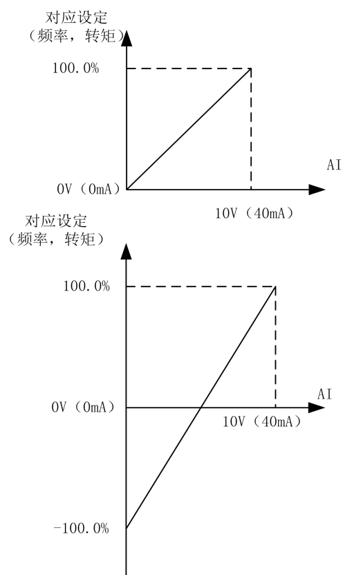
图 7-10 模拟给定与设定量的对应关系
