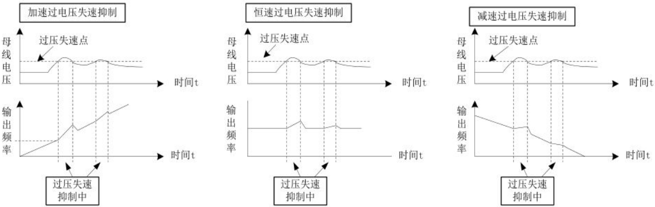
图 7-11 过压失速动作示意图
