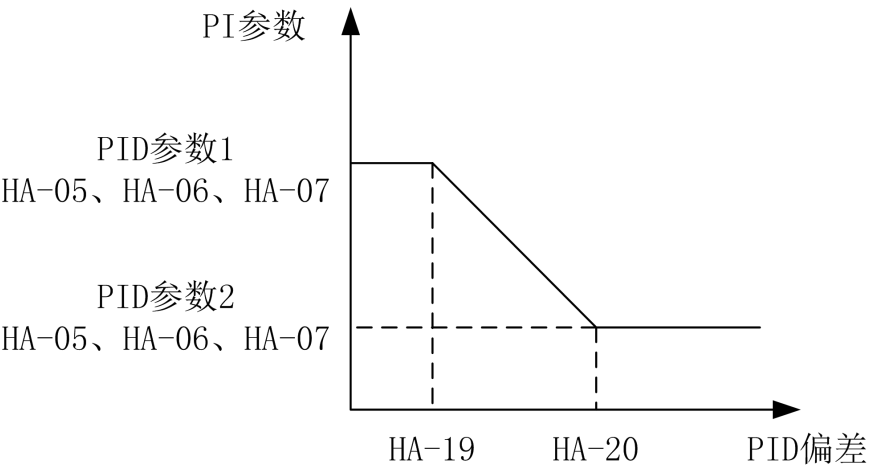
图 7-26 PID 参数切换
