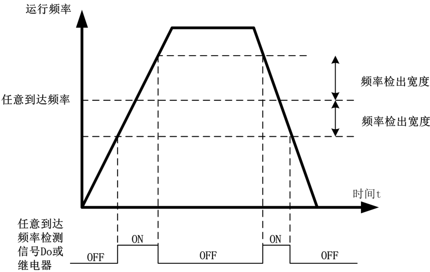
图 7-20 任意到达频率检测示意图
