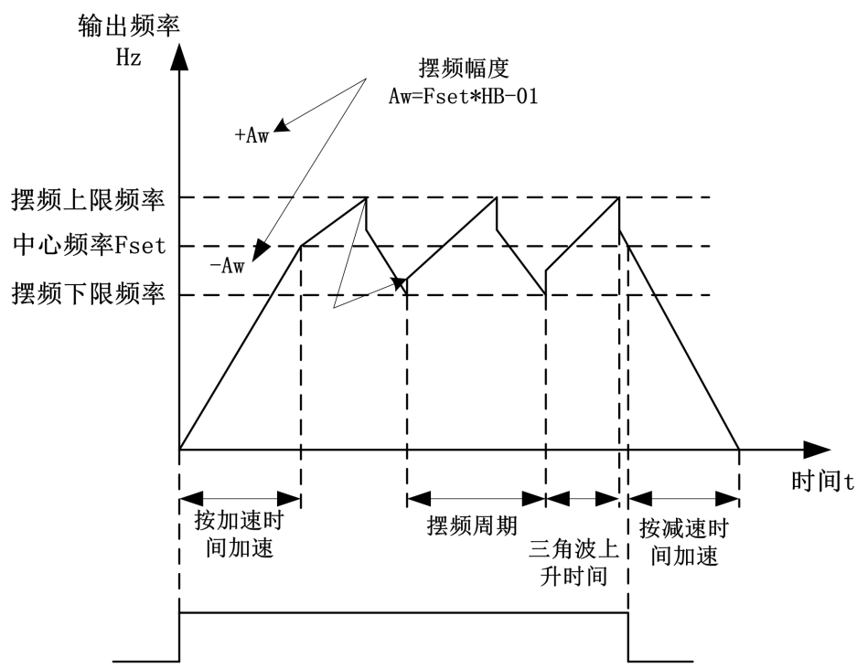
图 7-28 摆频工作示意图
