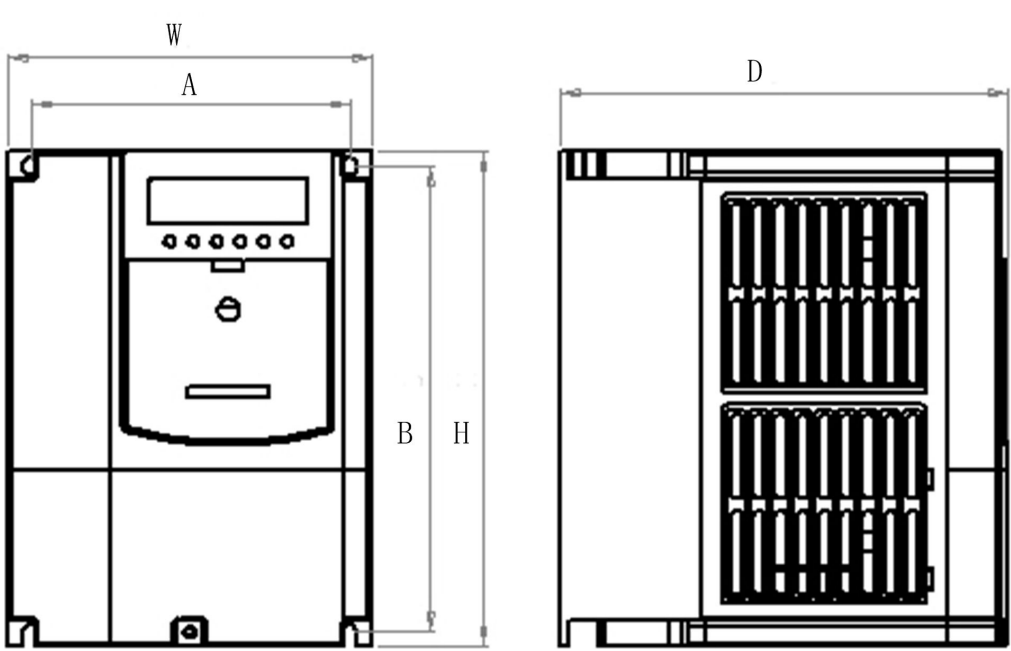
7.5kW 及以下机型的外形尺寸
