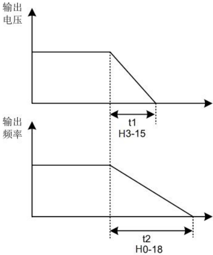
图 7-6 V/F 分离输出电压 / 频率独立减至 0
