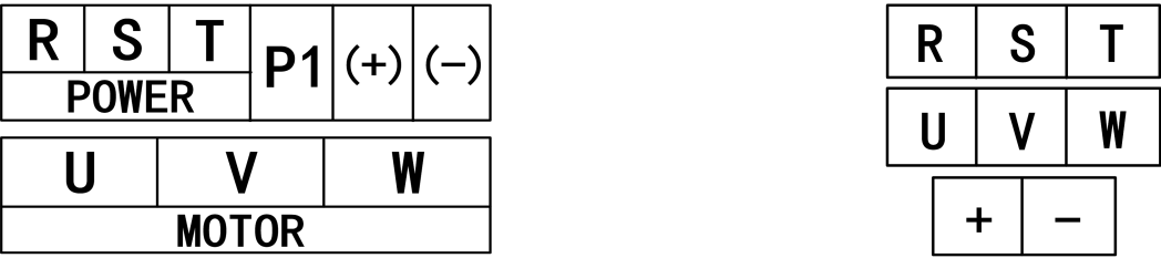
主回路接线端子图(160 ~ 400kW)
