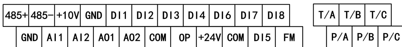
控制回路端子示意图
