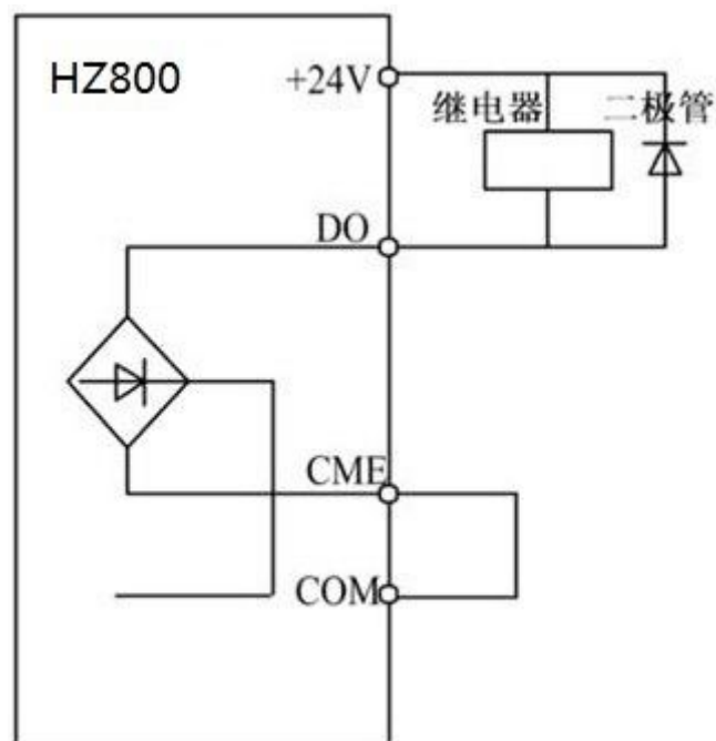
图 4-5 数字输出端子接线示意图
