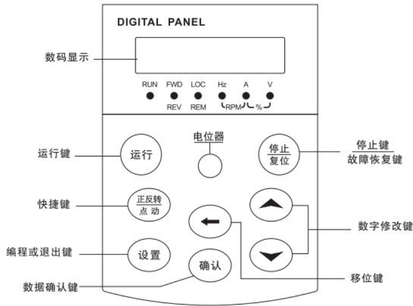
图 5-1 手持板图示
