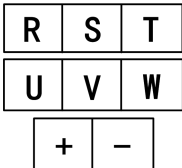
主回路接线端子图(400 ~ 630kW)
