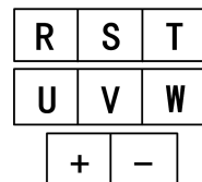
主回路接线端子图(400 ~ 630kW)
