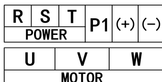
主回路接线端子图(185 ~ 350kW)
