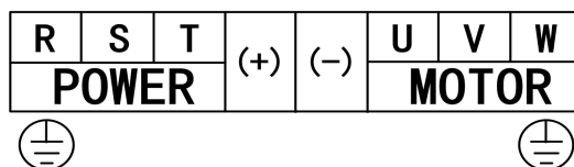
主回路接线端子图(55 ~ 160kW)
