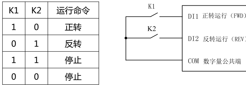
图 7-6 两线式模式 1
