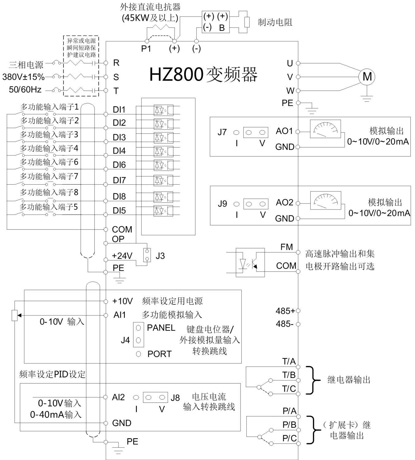
控制回路接线图
