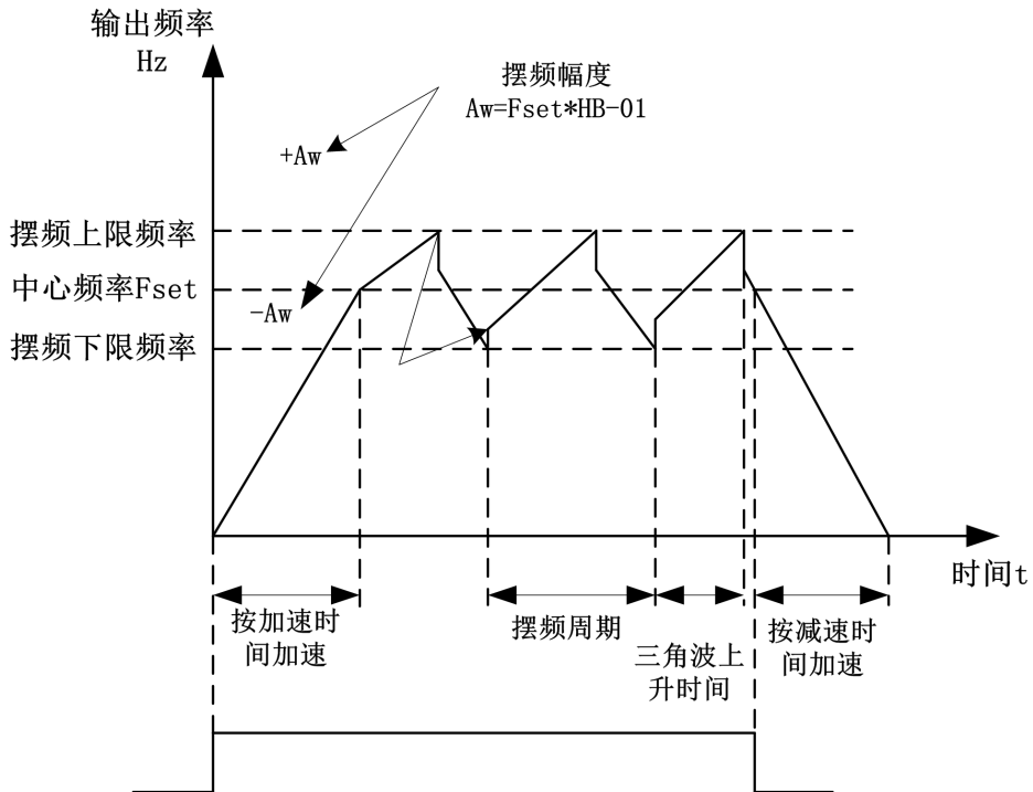
图 7-28 摆频工作示意图
