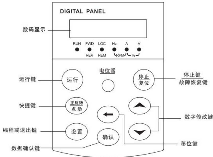
图 5-1 手持板图示
