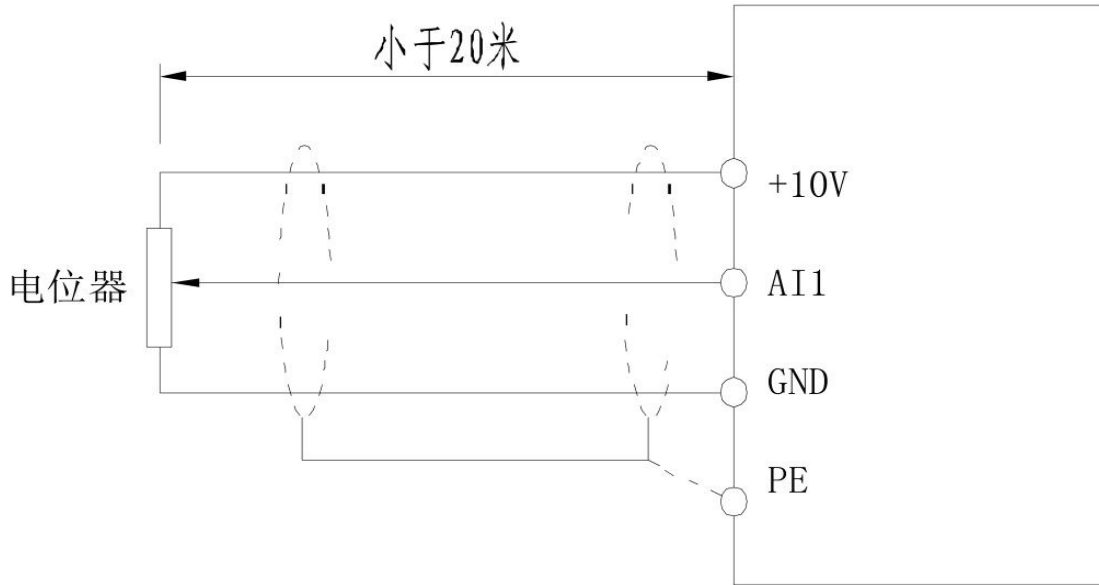
图 4-1 模拟量输入接线示意图
