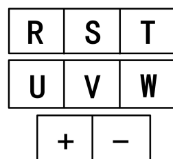
主回路接线端子图(500 ~ 710kW)
